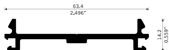
14350 MOLDURA UNIÓN Longitud: 6,10 m
