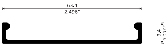
14349 TAPA PARA BÁSICO Longitud: 6,10 m
