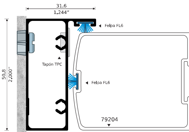
45844 BATIENTE 2" Longitud: 6.10 m
