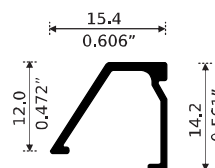
NUEVO 76371 JUNQUILLO BISELADO Longitud: 6.10 m
