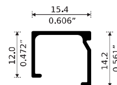
NUEVO 86370 JUNQUILLO RECTO Longitud: 6.10 m
