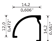
NUEVO 76372 JUNQUILLO CURVO Longitud: 6.10 m
