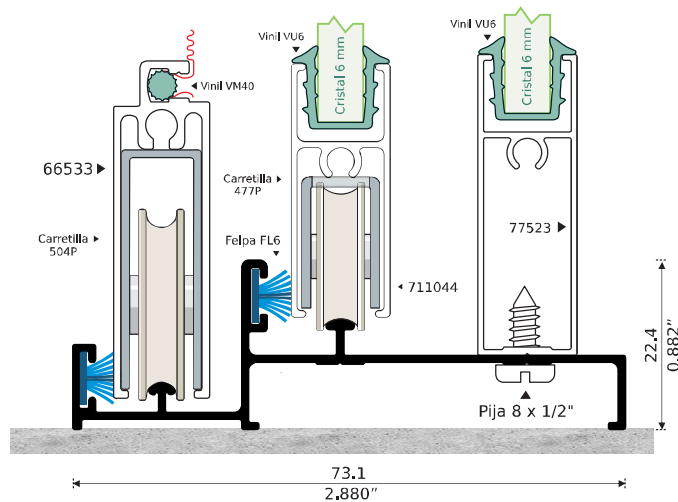
78371 RIEL CON MOSQUITERO INTERIOR Longitud: 6.10 m
