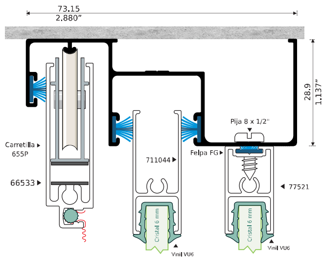
77819 PATENTE CONTRAMARCO CON MOSQUITERO CORREDIZO Longitud: 6,10 m
