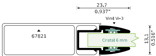
8270 PATENTE ADAPTADOR CURVO Longitud: 6,10 m
