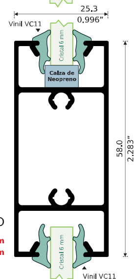
PATENTE 7837 INTERMEDIO Longitud: 6.10 m 7837-C 3.05 m
