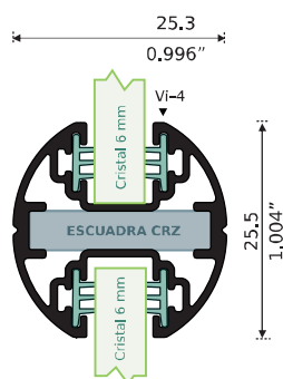
8271 PATENTE RETÍCULA DOBLE Longitud: 6.10 m
