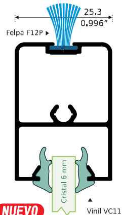
NUEVO 7834 CABEZAL Longitud: 6.10 m
