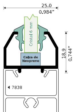
614702 NUEVO BASE CUADRÍCULA Longitud: 6.10 m
