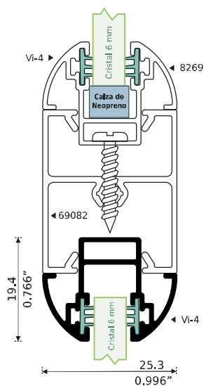
8269 PATENTE ADAPTADOR CURVO Longitud: 6.10 m
