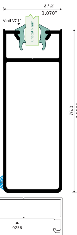
17847 CERCO CHAPA GRAN VISTA Longitud: 6.10 m 17847-C 4.60 m
