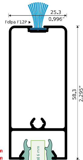
NUEVO 7838 ZOCLO CABEZAL Longitud: 6.10 m 7838-C 3.05 m
