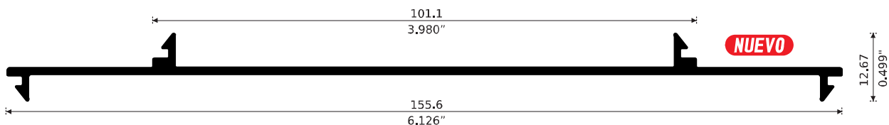
23609 MOLDURA UNIÓN Longitud 6.10 m
