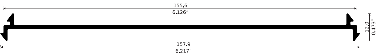
23618 MOLDURA UNIÓN Longitud: 6.10 m
