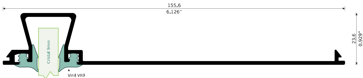
23615 TAPA BOLSA DESCENTRADA Longitud: 6.10 m
