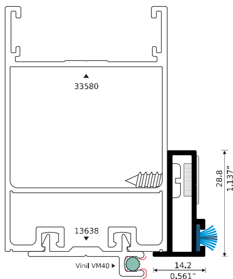
13639 ADAPTADOR CERCO Longitud: 6.10 m
