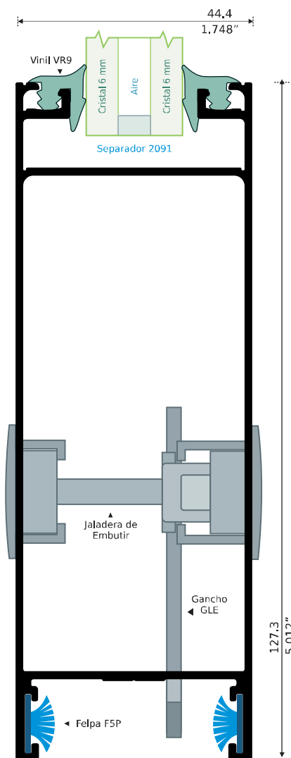
64083 CERCO CHAPA Longitud: 5,50 m
