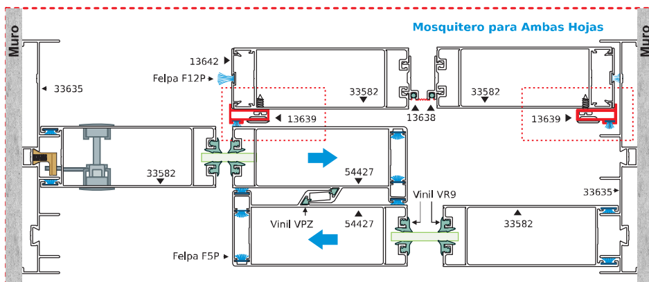
13639 ADAPTADOR CERCO Longitud: 6.10 m
