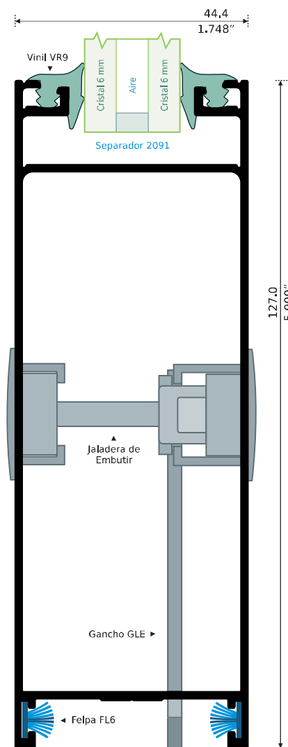
24083 PATENTE CERCO CHAPA Longitud: 5,50 m
