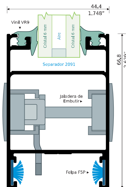
74083 CERCO CHAPA Longitud: 5,50 m
