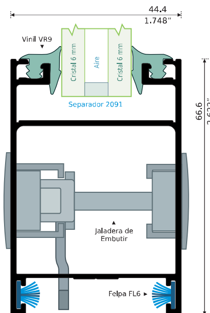
44083 CERCO CHAPA VENTANA Longitud: 5,50 m
