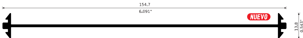
23630 MOLDURA UNIÓN Longitud 6.10 m
