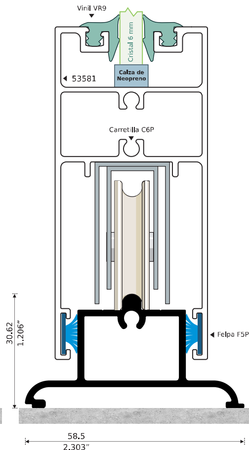
15230 PATENTE RIEL Y CABEZAL Longitud: 6.10 m
