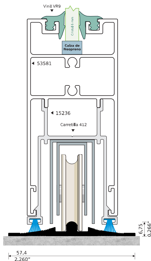
15231 PATENTE RIEL SENCILLO Longitud: 6.10 m
