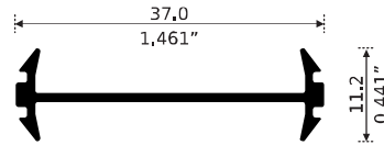
12623 MOLDURA UNION Longitud: 6.10 m
