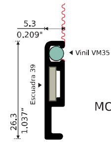
5173 MOSQUITERO Longitud: 6.10 m
