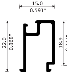
NUEVO 12609 JUNQUILLO Longitud: 6.10 m
