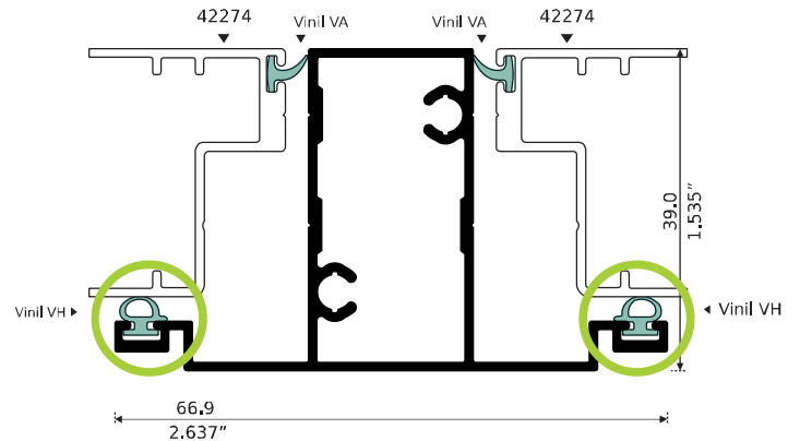
42275 NUEVO INTERMEDIO Longitud: 6,10 m
