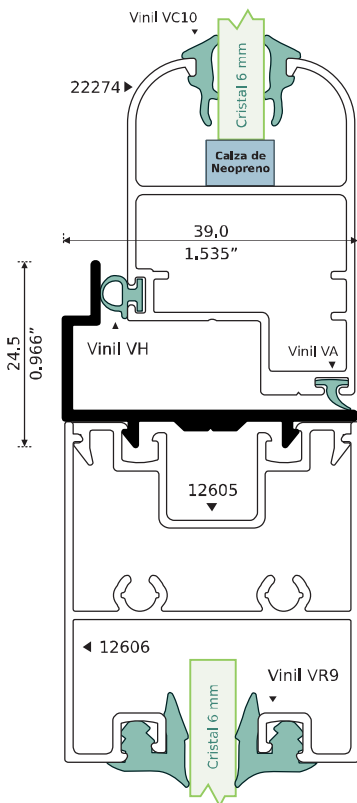
13609 ADAPTADOR FIJO BATIENTE Longitud: 6.10 m
