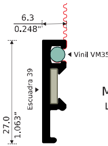
13609 ADAPTADOR FIJO BATIENTE Longitud: 6.10 m
