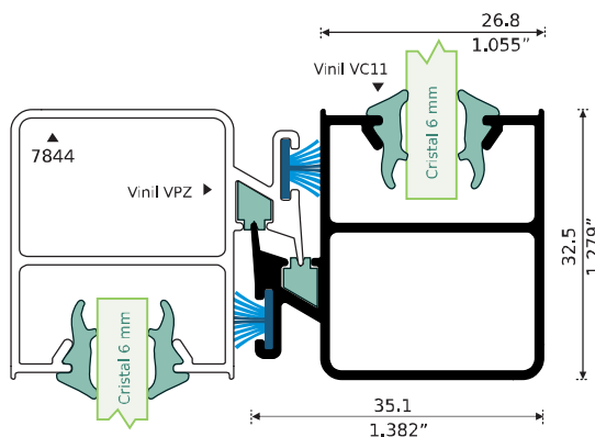
PATENTE 7844 TRASLAPE VENTANA Longitud: 6.10 m
