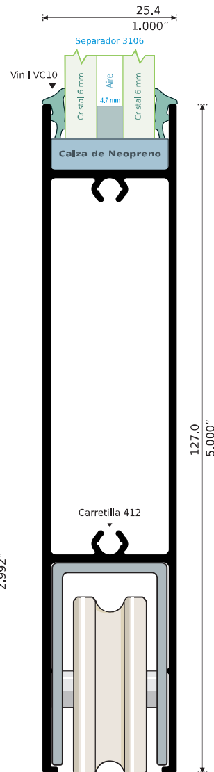
19959 NUEVO ZOCLO PUERTA 5" Longitud: 6,10 m
