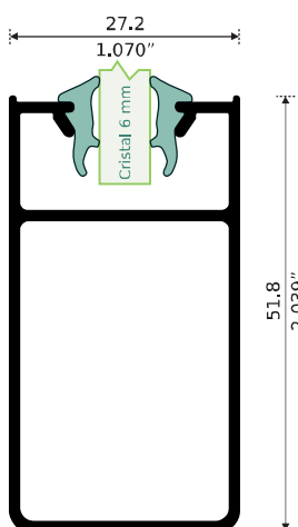
7843 CERCO Longitud: 6.10 m
