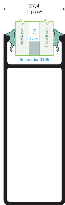
19964 CERCO CHAPA GRAN VISTA Longitud: 6,10 m
