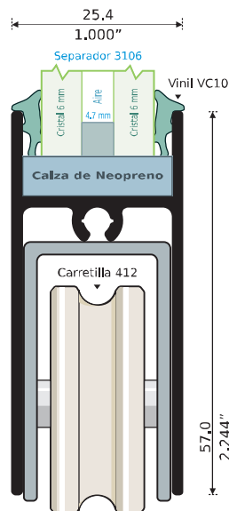
9960 CABEZAL Y ZOCLO Longitud: 6,10 m
