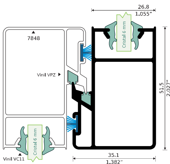
PATENTE 7848 TRASLAPE PUERTA Longitud: 4.60 m 7848-L 6.10 m
