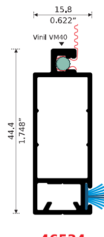
46534 MOSQUITERO ARMADO A 45° Y A 90° Longitud: 6.10 m
