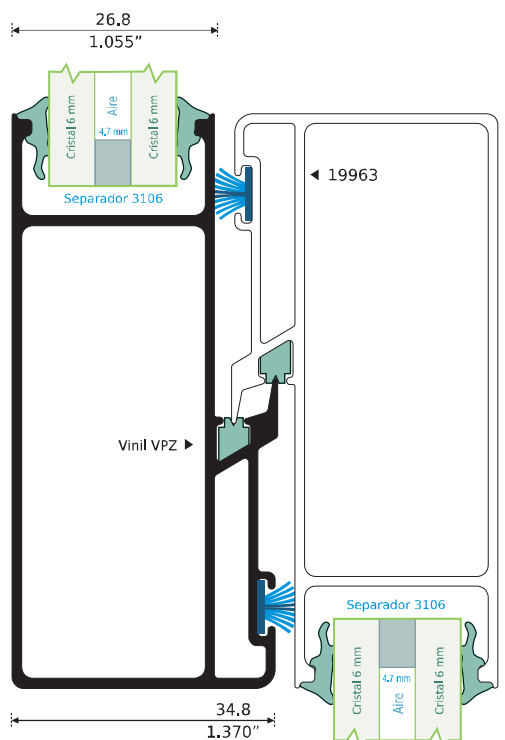
19963 TRASLAPE GRAN VISTA Longitud: 6,10 m
