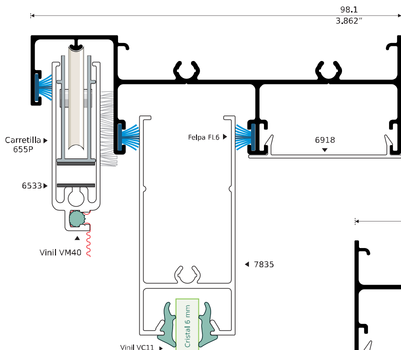
47862 PATENTE CONTRAMARCO CON MOSQUITERO CORREDIZO COLGANTE Longitud: 6,10 m
