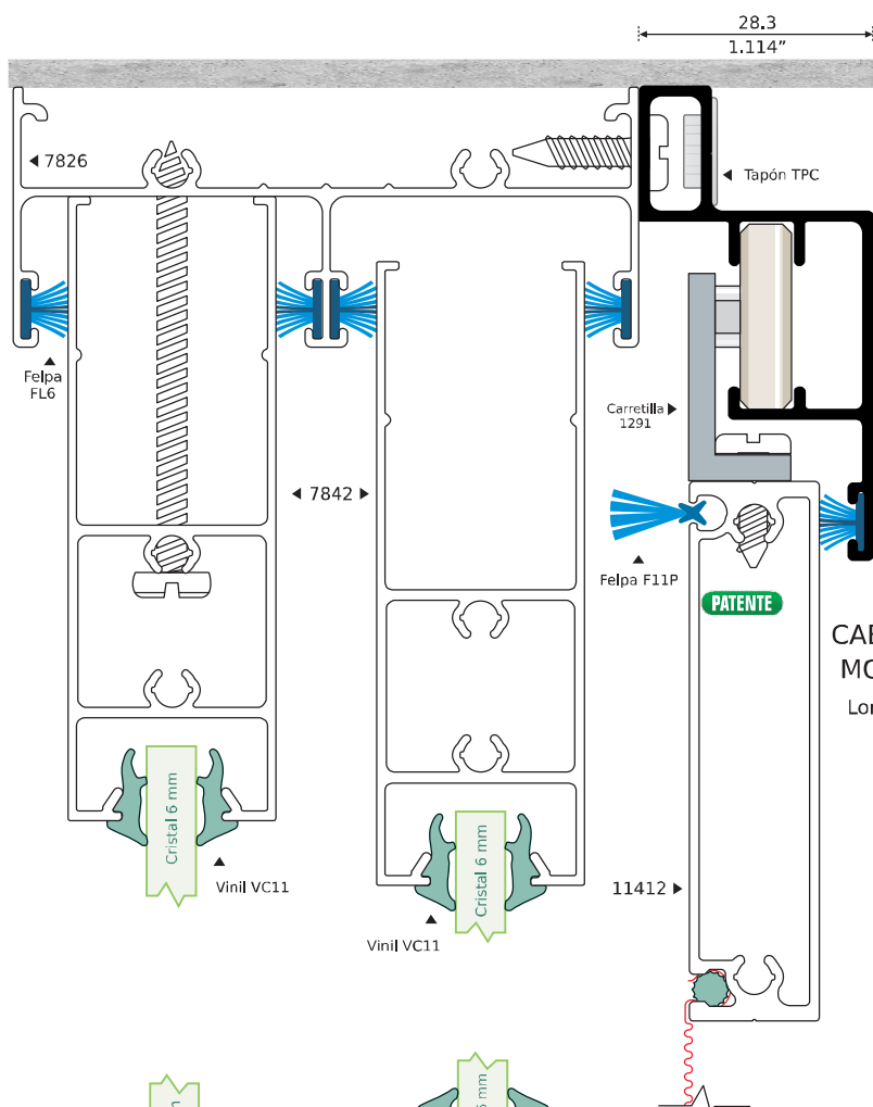
11412 MOSQUITERO Longitud: 6.10 m
