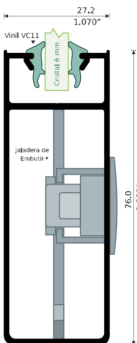
17847 CERCO CHAPA GRAN VISTA Longitud: 6.10 m 17847-C 4.60 m
