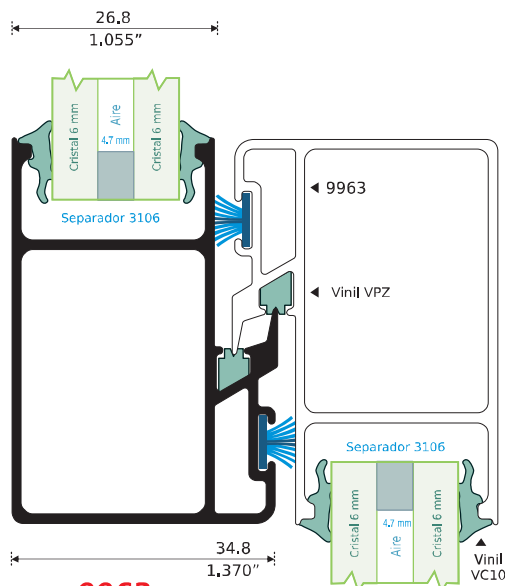
9963 TRASLAPE Longitud: 6,10 m
