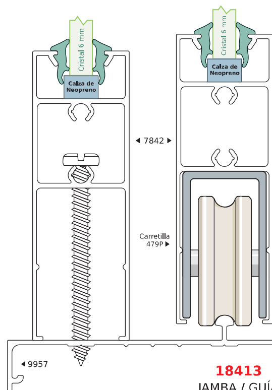
18413DREN Drenes cada 60 cm
