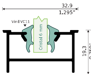
8681 PATENTE CERCO FIJO Longitud: 6.10 m
