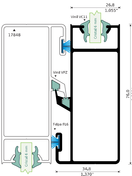
PATENTE 17848 TRASLAPE GRAN VISTA Longitud: 6.10 m
