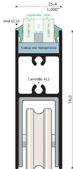
9959 ZOCLO PUERTA Longitud: 6,10 m
