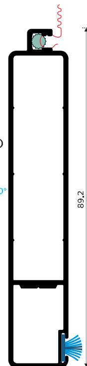
16533 MOSQUITERO HORIZONTAL Longitud: 6.10 m
