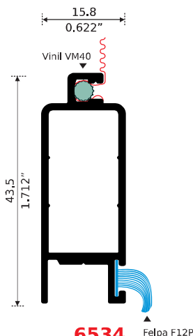
6534 MOSQUITERO VERTICAL Longitud: 4.60 m 6534-L 6.10 m
