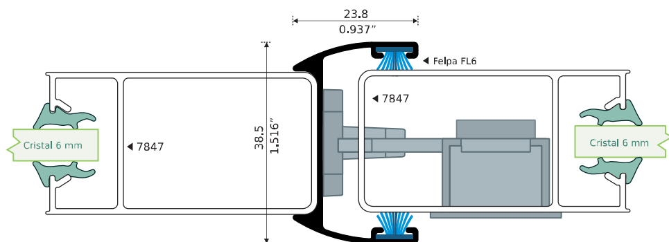
7851 PATENTE ADAPTADOR OXXO
