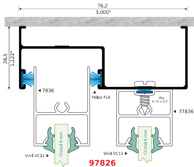
97826 CONTRAMARCO SIN VENAS
