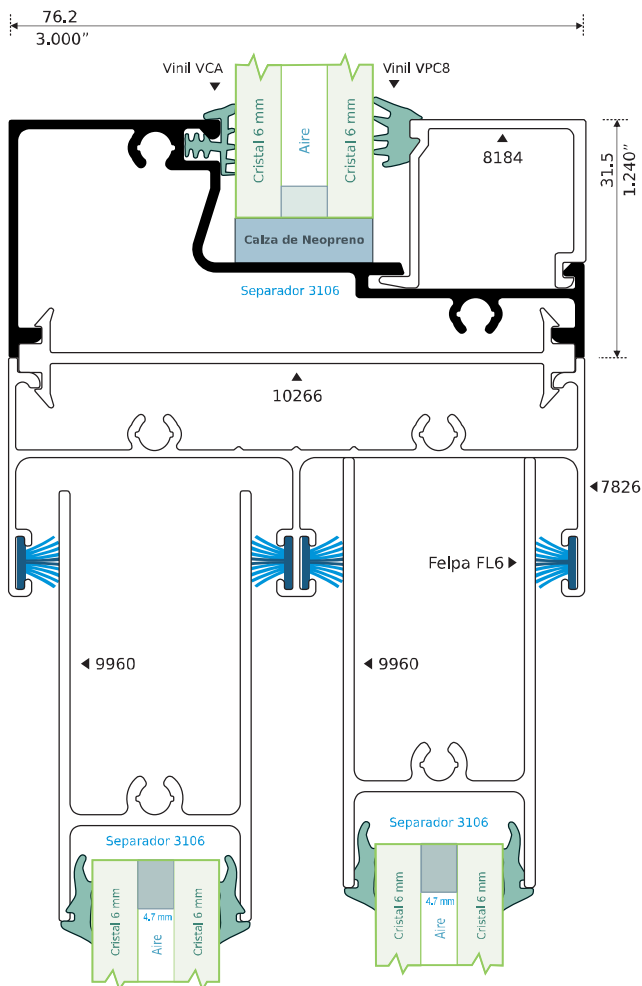
28183 ESCALONADO Longitud: 6.10 m
