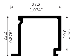
8184 JUNQUILLO Longitud: 6.10 m
