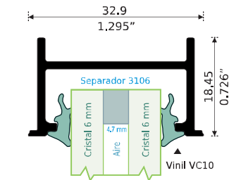
9965 CERCO FIJO Longitud: 6,10 m
