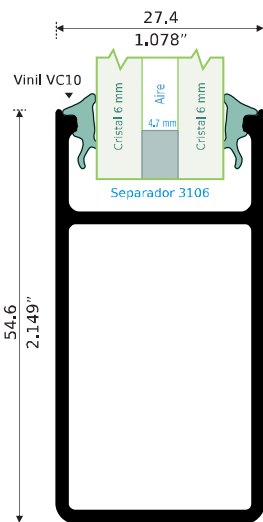
9964 CERCO CHAPA Longitud: 6,10 m
