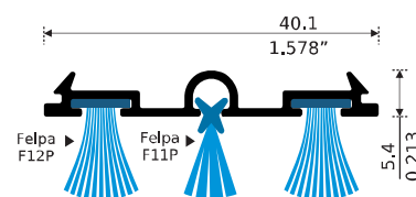
19188 SELLO DE HERMETICIDAD 3 FELPAS Longitud: 6.10 m 19188-C 3.05 m
