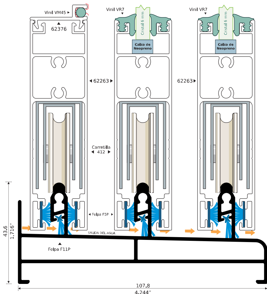
48407 RIEL Y CABEZAL TRIPLE
