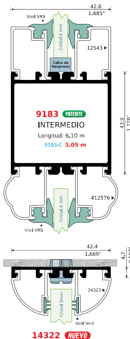
14322 NUEVO PORTA JUNQUILLOS Longitud: 6.10 m
