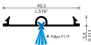
49188 SELLO DE HERMETICIDAD 1 FELPA Longitud: 6.10 m
